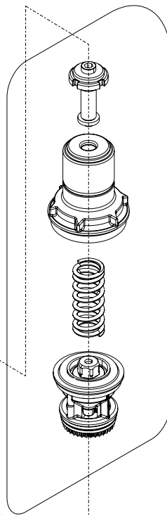
Druckminderer YSK233200903
